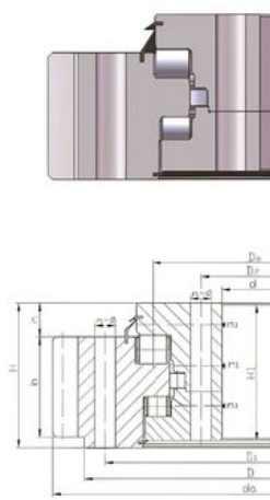
外齿式 Outer teeth
