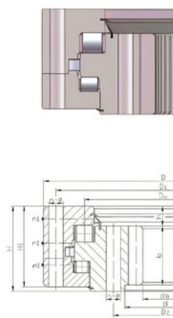
内齿式 Inner teeth
