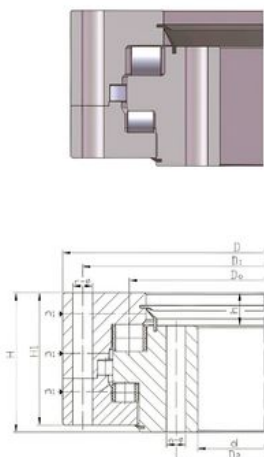
无齿式 No teeth
